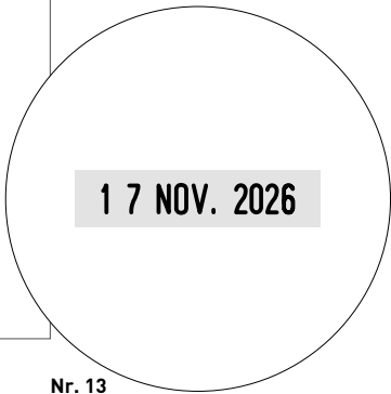
Nr. 13 Ø 47mm Max. dimensioni piastra di testo 4mm | Altezza caratteri data
