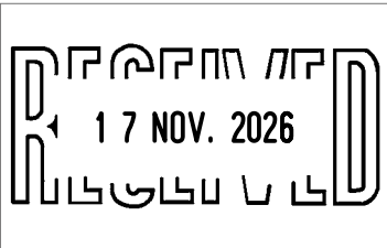
2210L - 47 x 30mm | Max. dimensioni piastra di testo 4mm | Altezza caratteri data Disponibile in lingua inglese, altre lingue su richiesta
